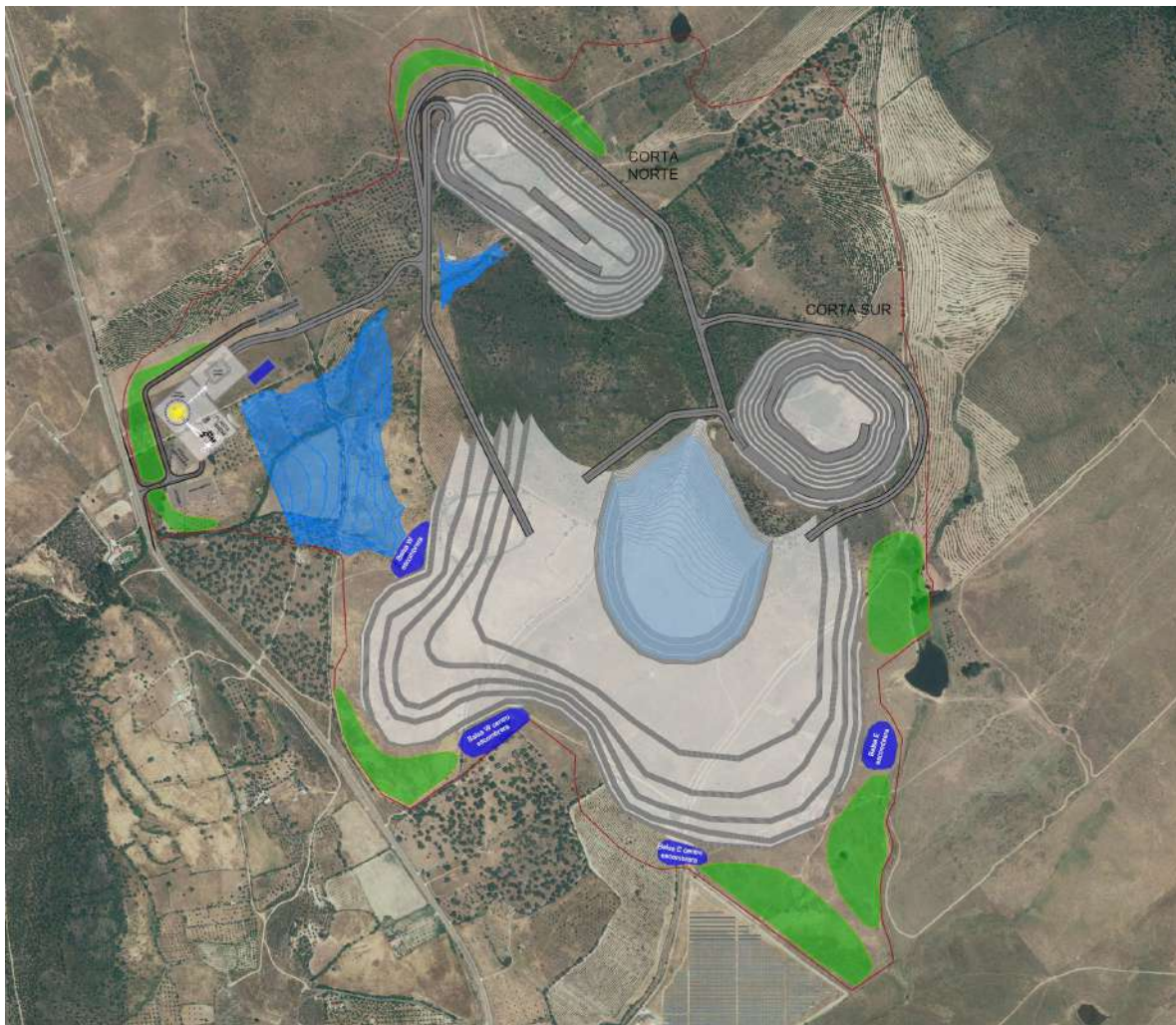
Ilustración 5: ocupación directa y envolvente de la explotación
